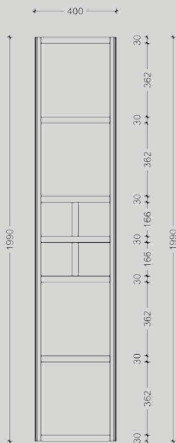
κύρια όψη
